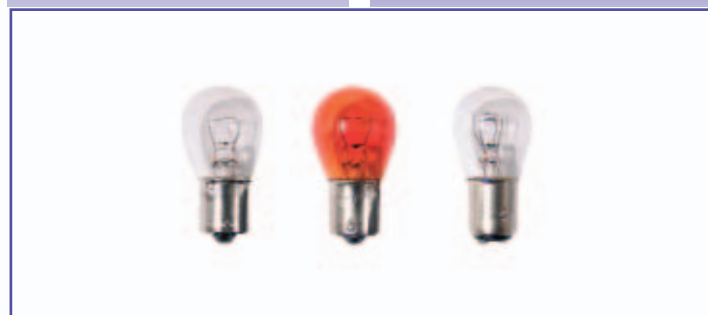
IZZÓ 12V 10W BA15 STARLIGHT 4854-TUN 15,-Ft
