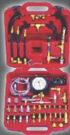
94661-FRC ÜZEMANYAGRENDSZER NYOMÁSMÉRŐ KÉSZLET
